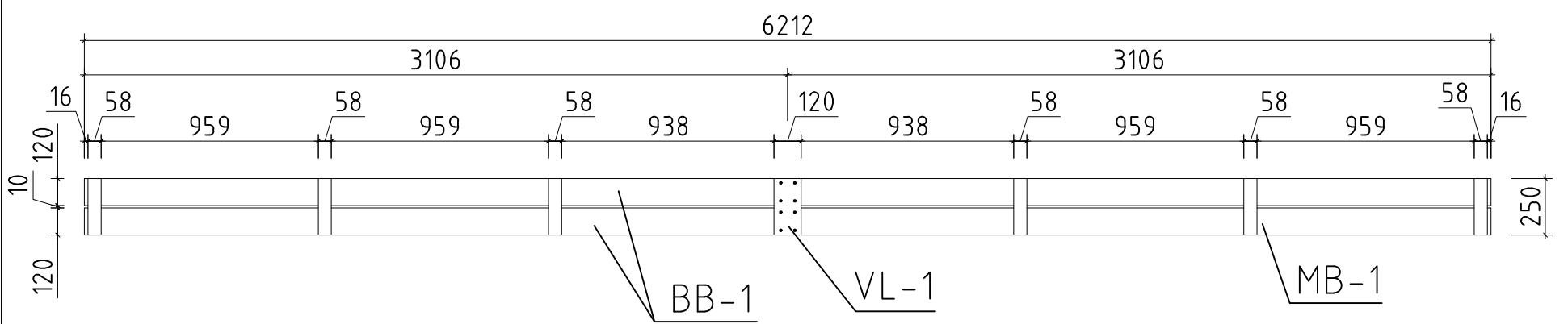
DACHBLENDEN 1 - PARAPET 1
