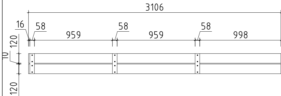
DACHBLENDEN 1a - PARAPET 1a
