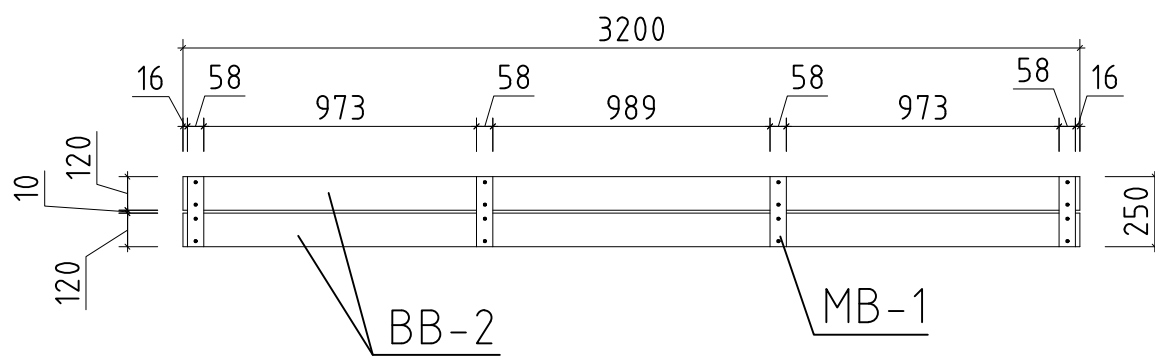
DACHBLENDEN 2 - PARAPET 2
