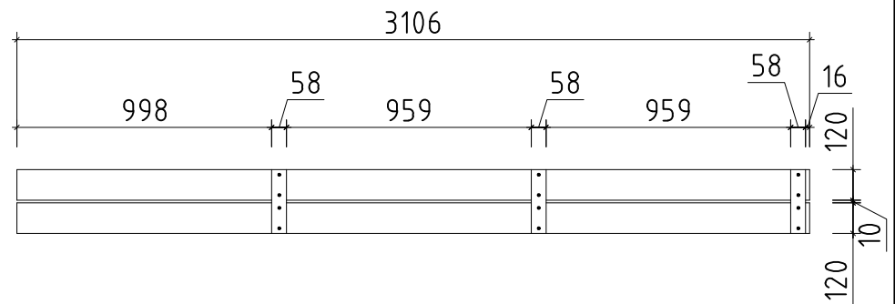
DACHBLENDEN 1b - PARAPET 1b
